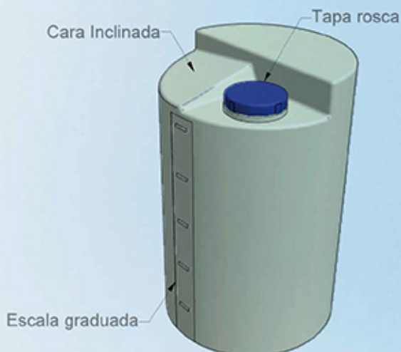
Vista perspectiva
