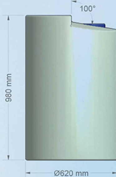
Vista lateral
