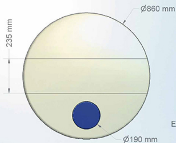
Vista superior
